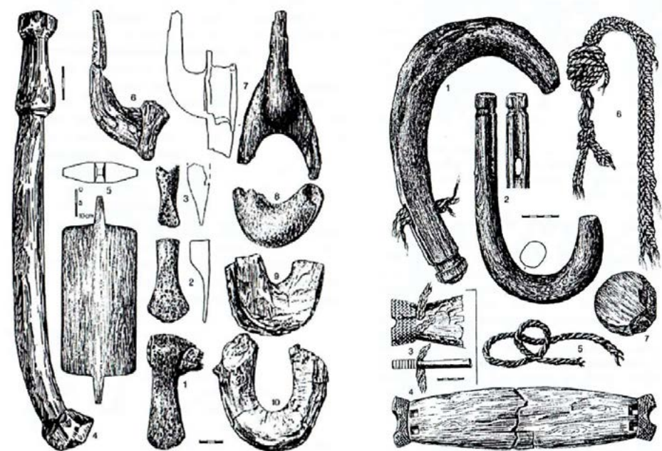
Drevininko įrankiai ir geinio fragmentai. Araišų ežero gyvenvietė. IX–X a. Apals J., Senākiemeža dravniecības darbarīku atradumi Latvijā, Arheoloģija un etnografija , t. 20: Pētījumi par Kurzemi un Zemgali, Rīga, 2000, p. 15, 3. att.
